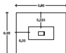
ΚΑΤΟΨΗ ΘΕΜΕΛΙΟΥ
